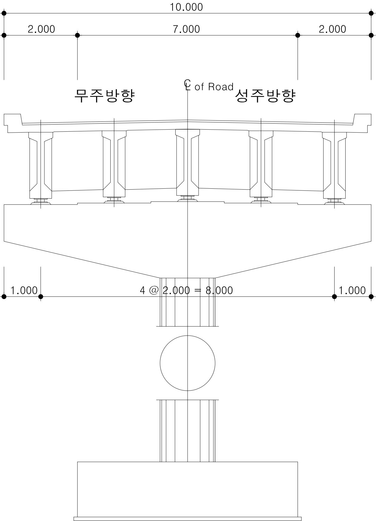
【그림 1.2】 횡단면도
